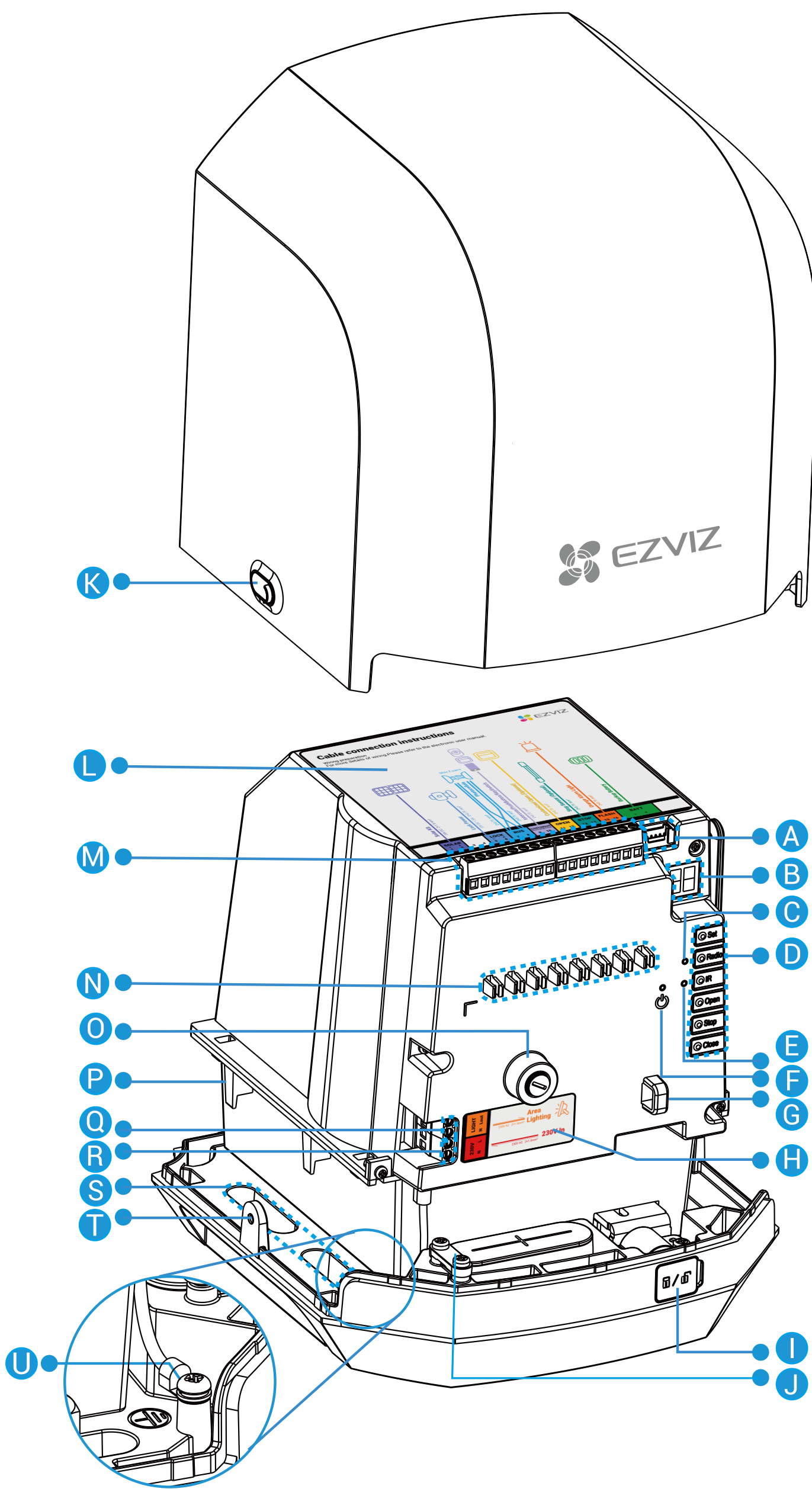
Προβολή μπροστά
