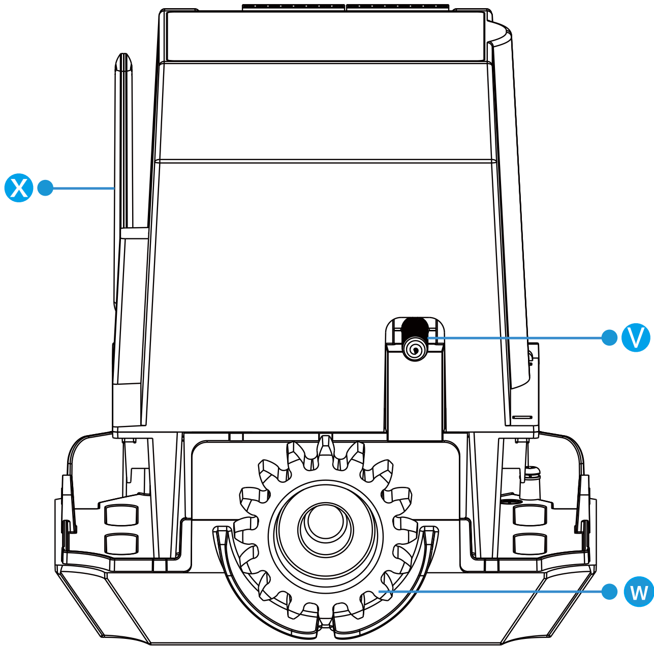
Πίσω όψη
