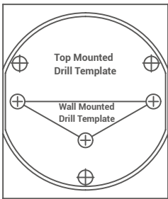
Πρότυπο διάτρησης (×1)
