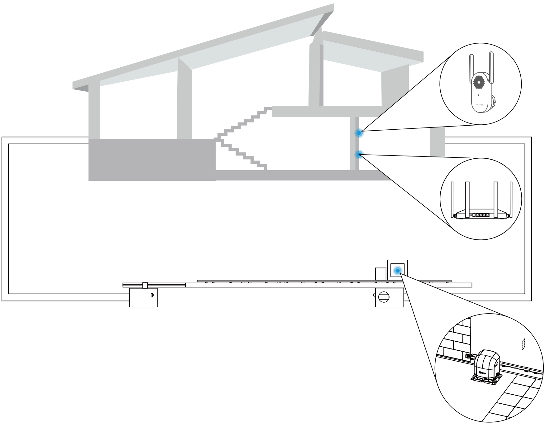
Τοπολογία ασύρματης επικοινωνίας
